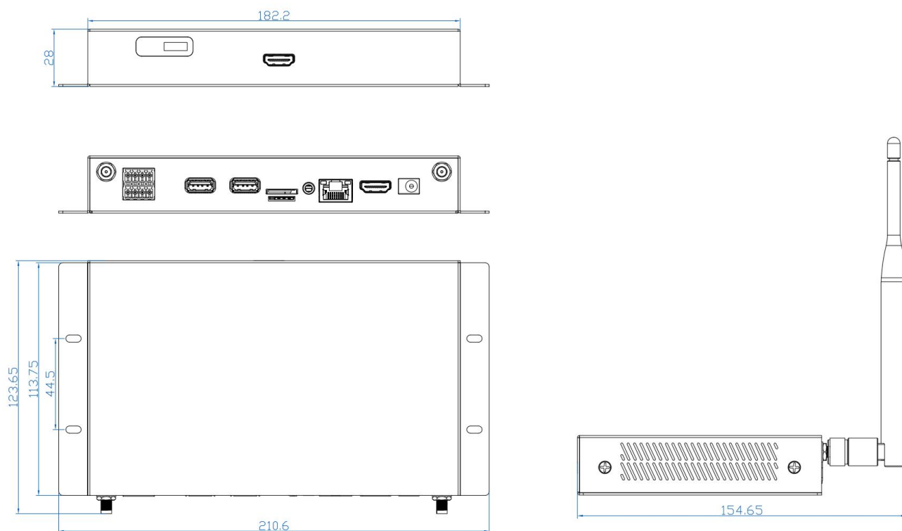
侧面接口尺寸 (装盒)
